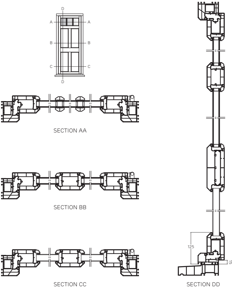
The English Door Ballingdon Door
